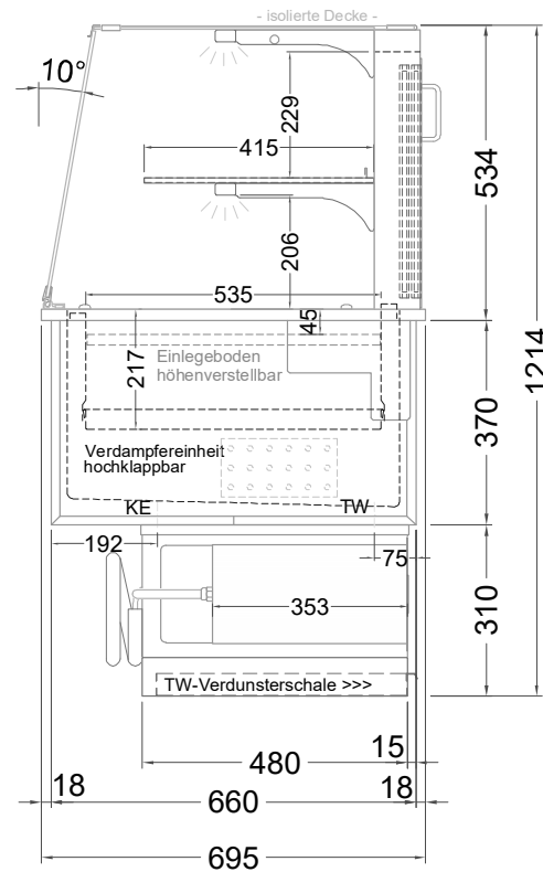
(Seitenansicht)
