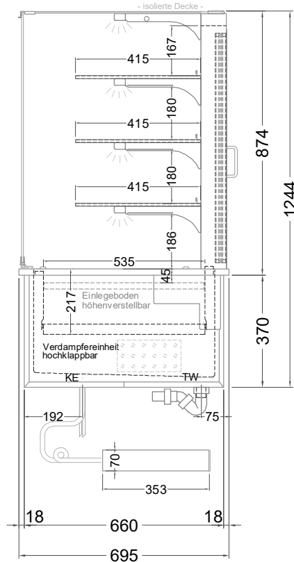
(Seitenansicht)
