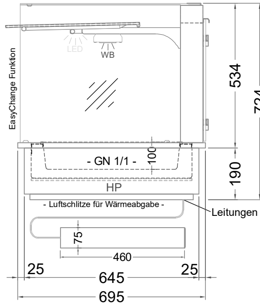
(Seitenansicht)
