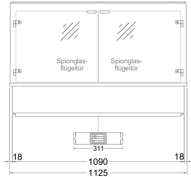
(Bedienseite)
