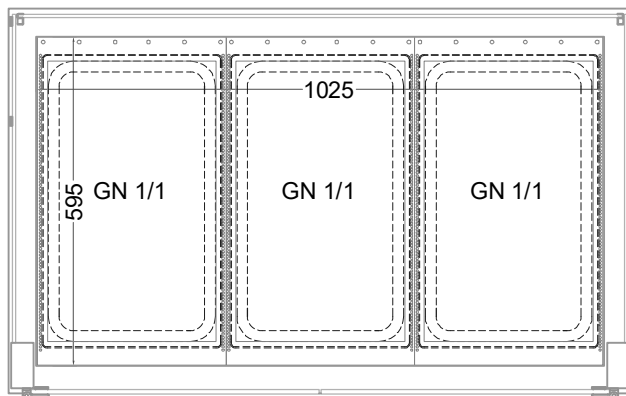
(Grundriss)
