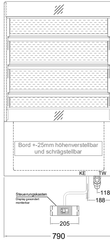
(Vorderseite)
