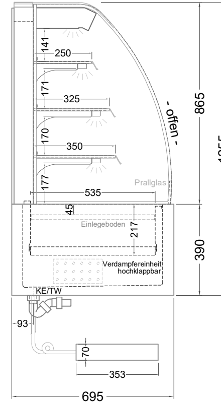
(Seitenansicht)
