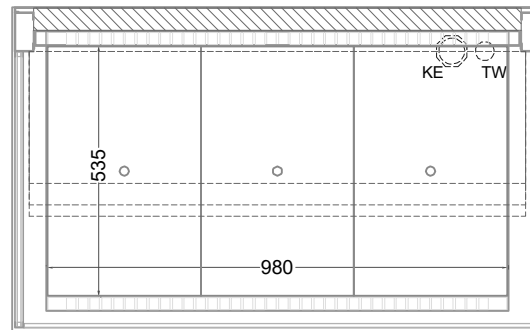
(Grundriss)
