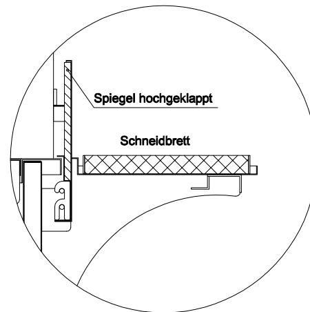
(Detail Spiegelsystem)
