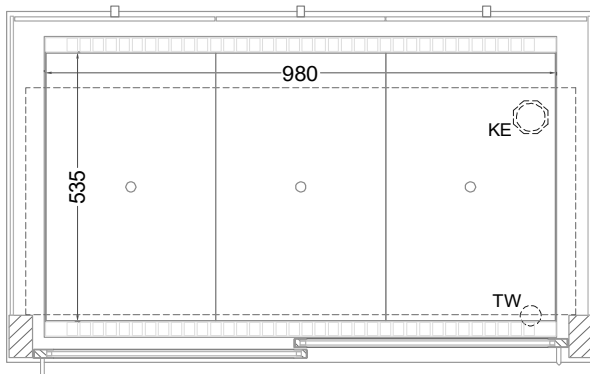
(Grundriss)
