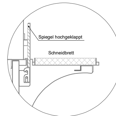
(Detail Spiegelsystem)
