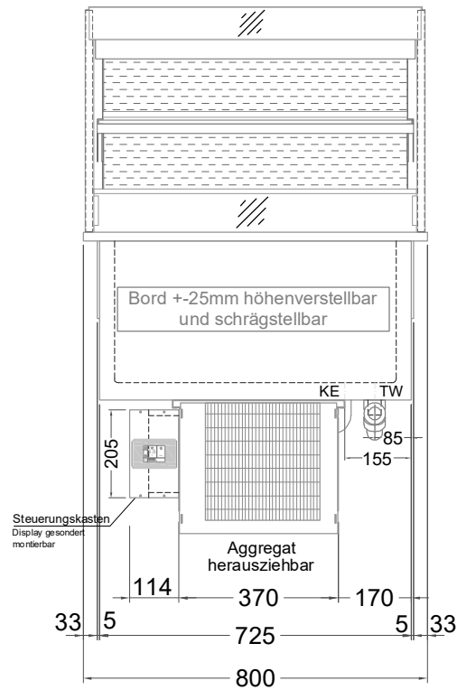
(Grundriss)
