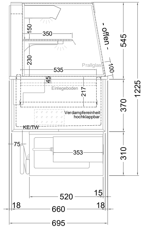
(Seitenansicht)
