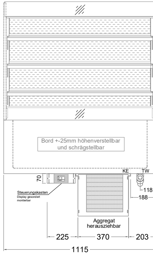
(Vorderseite)
