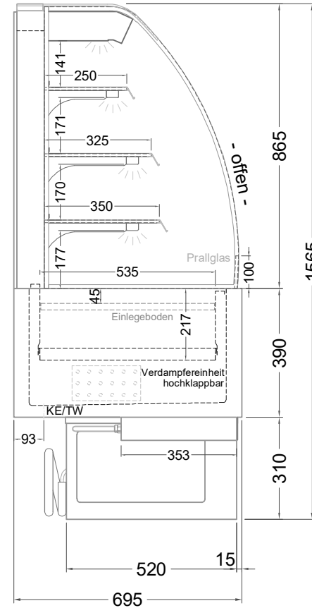
(Seitenansicht)
