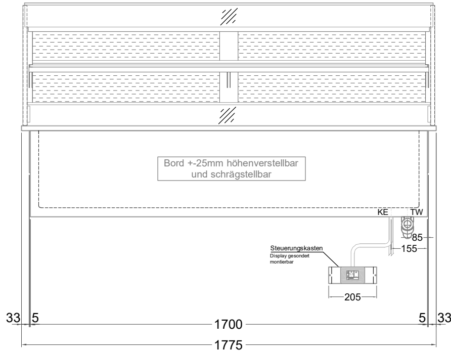
(Vorderseite)
