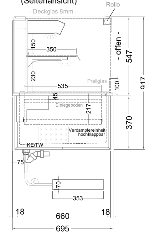
(Seitenansicht)
