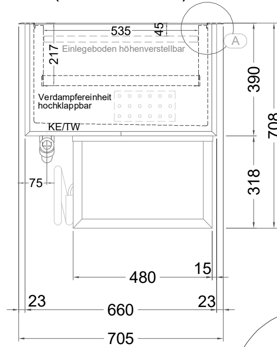
(Seitenansicht)
