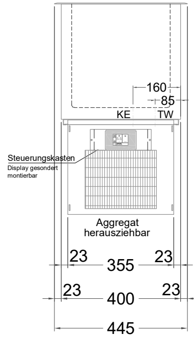
(Grundriss)
