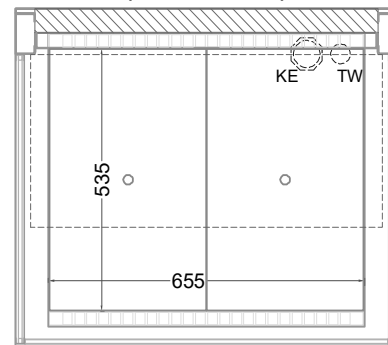
(Grundriss)
