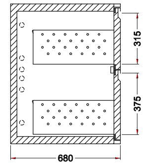
Schnitt L1
