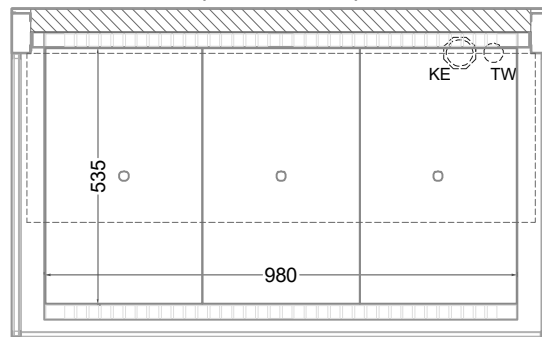
(Grundriss)
