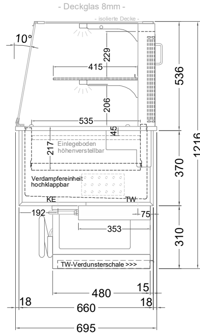
(Seitenansicht)
