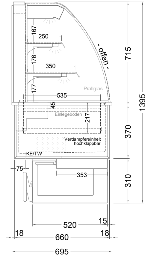
(Seitenansicht)
