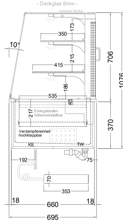
(Seitenansicht)
