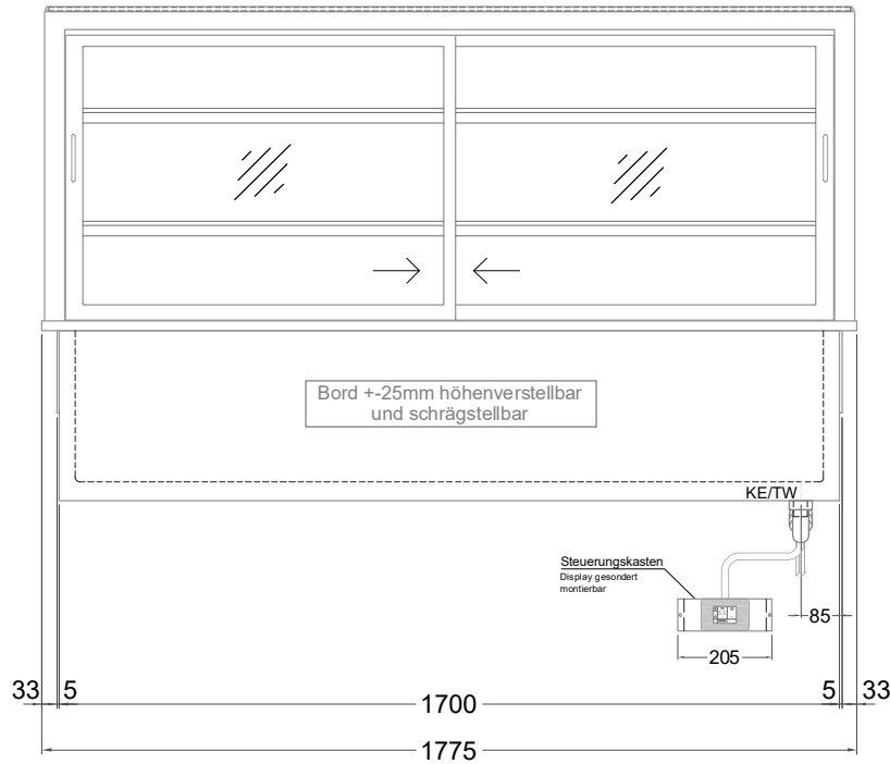
(Bedienseite)
