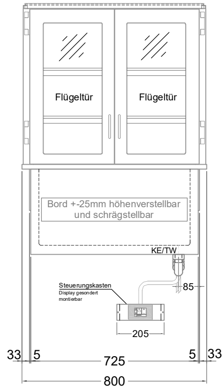
(Bedienseite)
