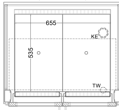
(Grundriss)
