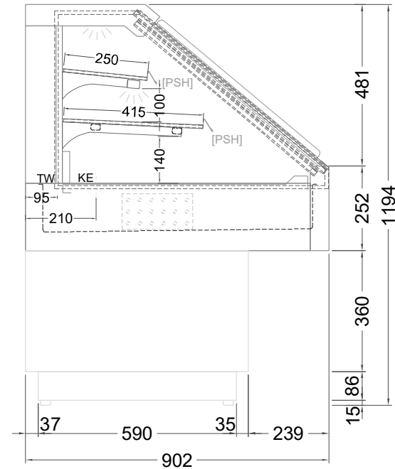
(Seitenansicht)
