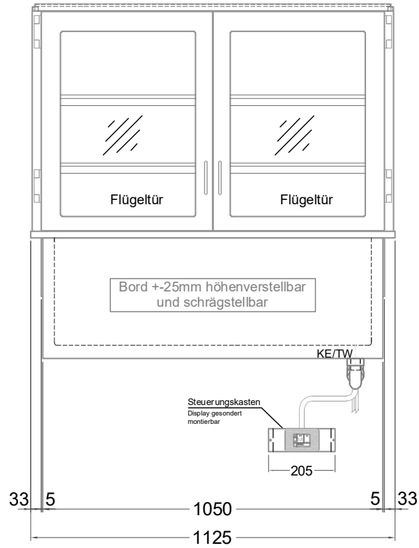
(Bedienseite)
