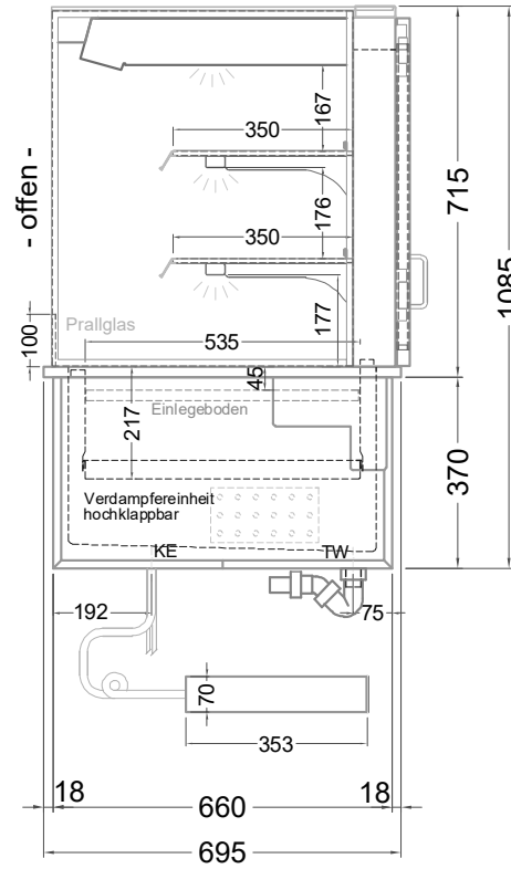
(Seitenansicht)
