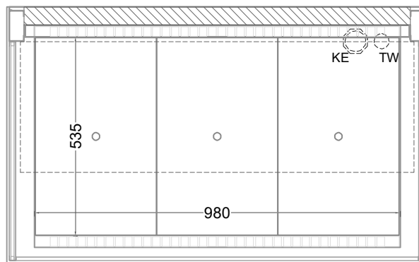
(Grundriss)
