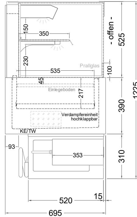
(Seitenansicht)
