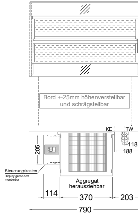
(Vorderseite)
