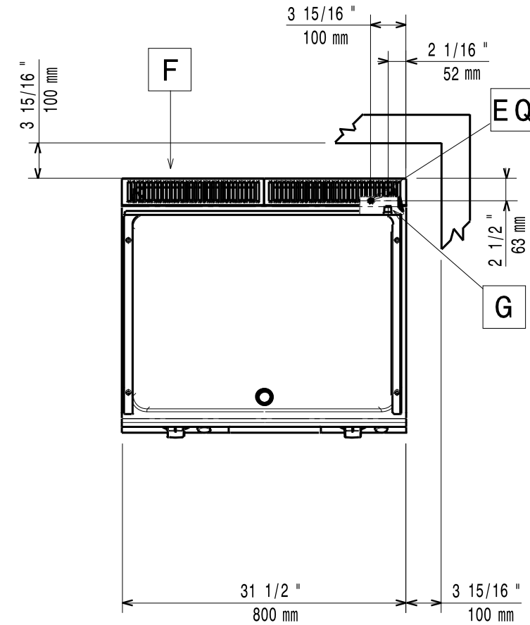
[Draufsicht]
