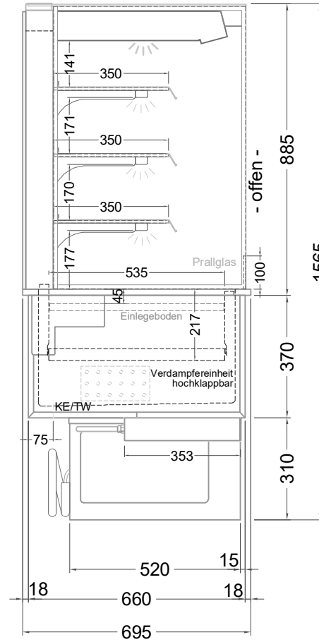
(Seitenansicht)
