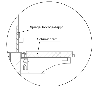
(Detail Spiegelsystem)
