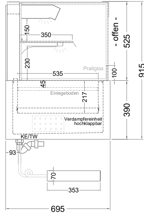
(Seitenansicht)
