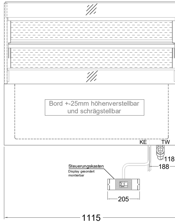
(Vorderseite)
