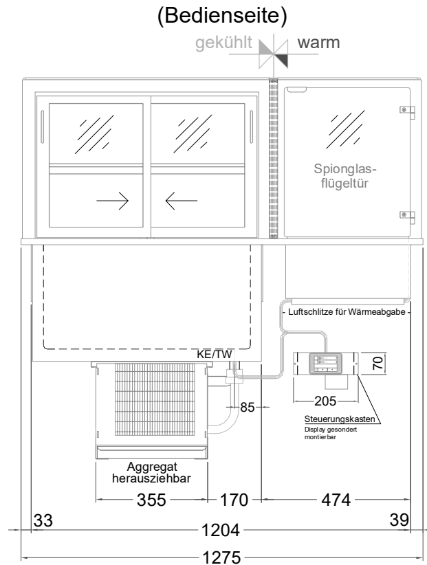
(Grundriss)
