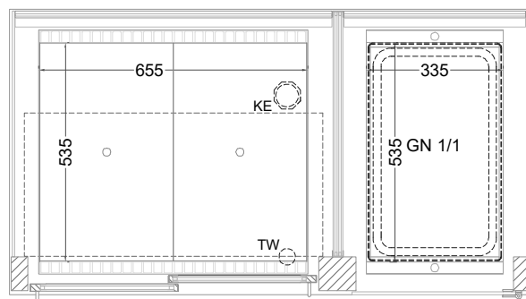
(Grundriss)
