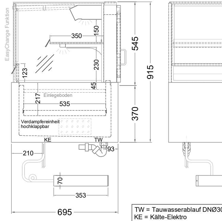
(Seitenansicht)
