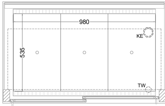
(Grundriss)
