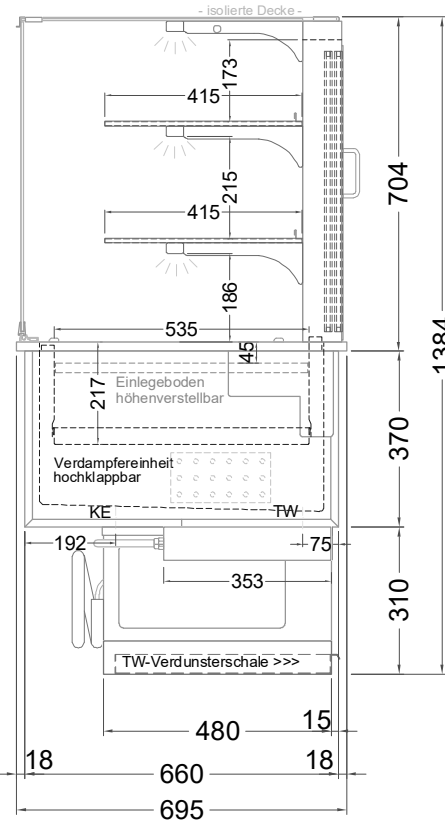
(Seitenansicht)
