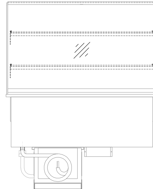
(Kundenseite)
