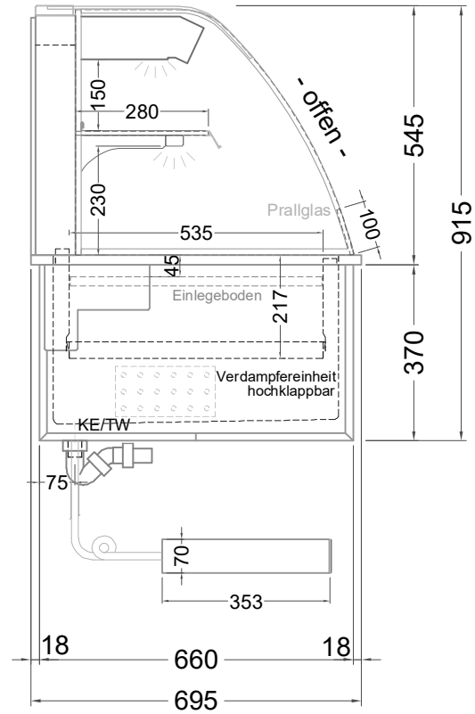
(Seitenansicht)
