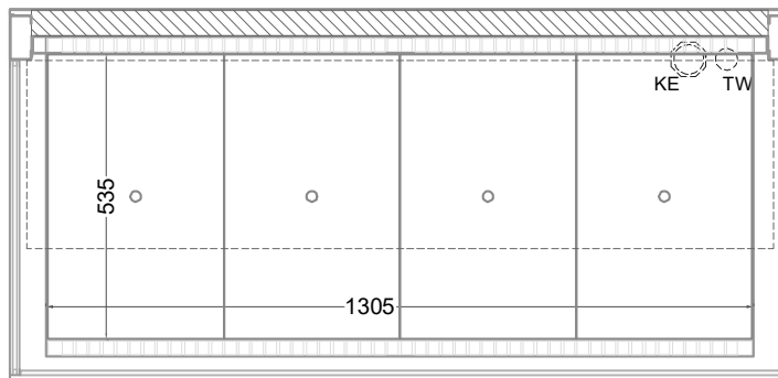
(Grundriss)
