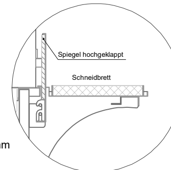
(Detail Spiegelsystem)
