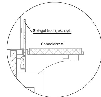
(Detail Spiegelsystem)
