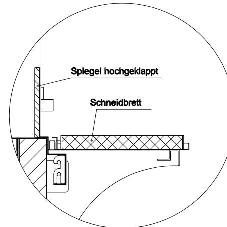
(Detail Spiegelsystem)
