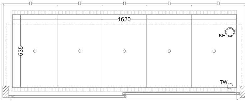
(Grundriss)
