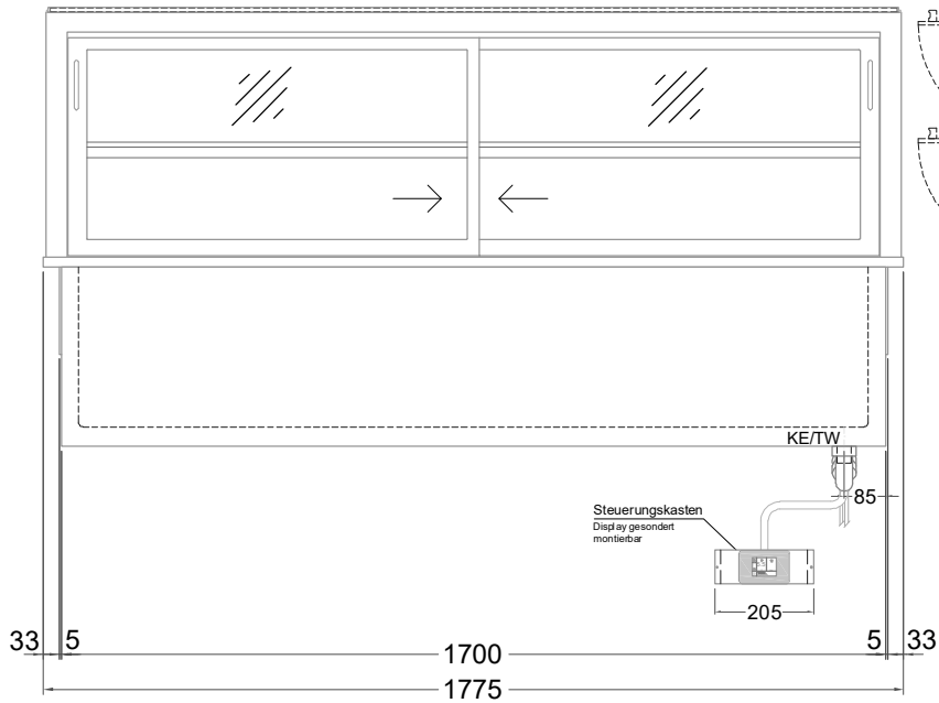
(Bedienseite)
