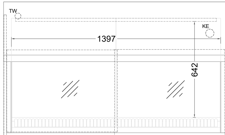
(Grundriss)
