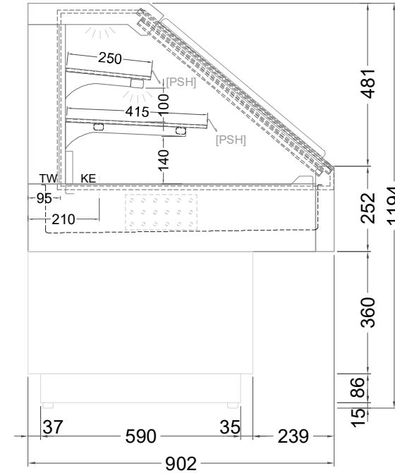
(Seitenansicht)
