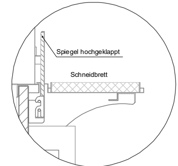
(Detail Spiegelsystem)
