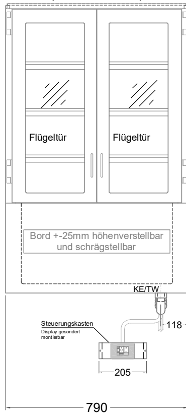
(Bedienseite)
