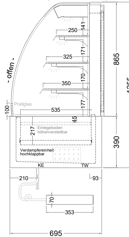
(Seitenansicht)
