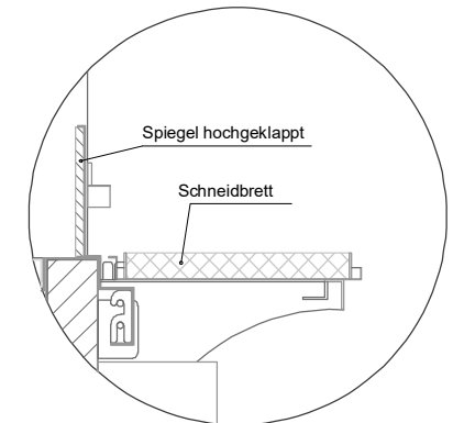
(Detail Spiegelsystem)
