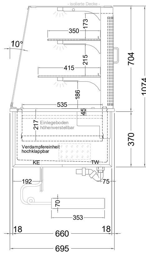
(Seitenansicht)
