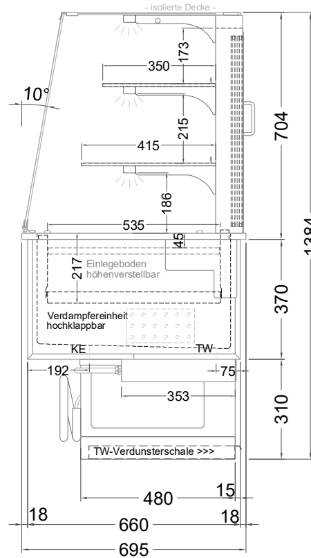
(Seitenansicht)
