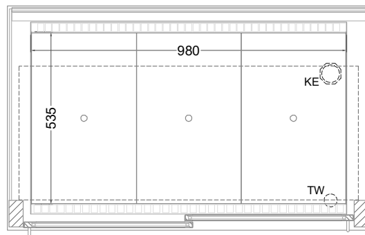
(Grundriss)
