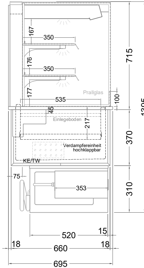
(Seitenansicht)
