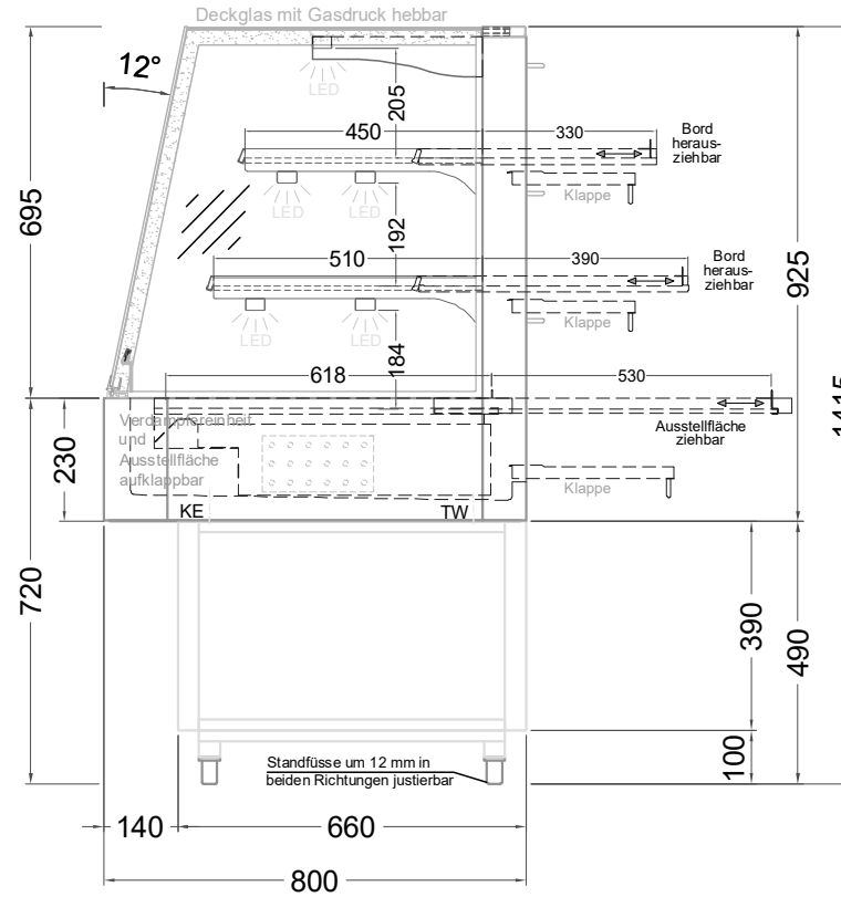
(Seitenansicht)
