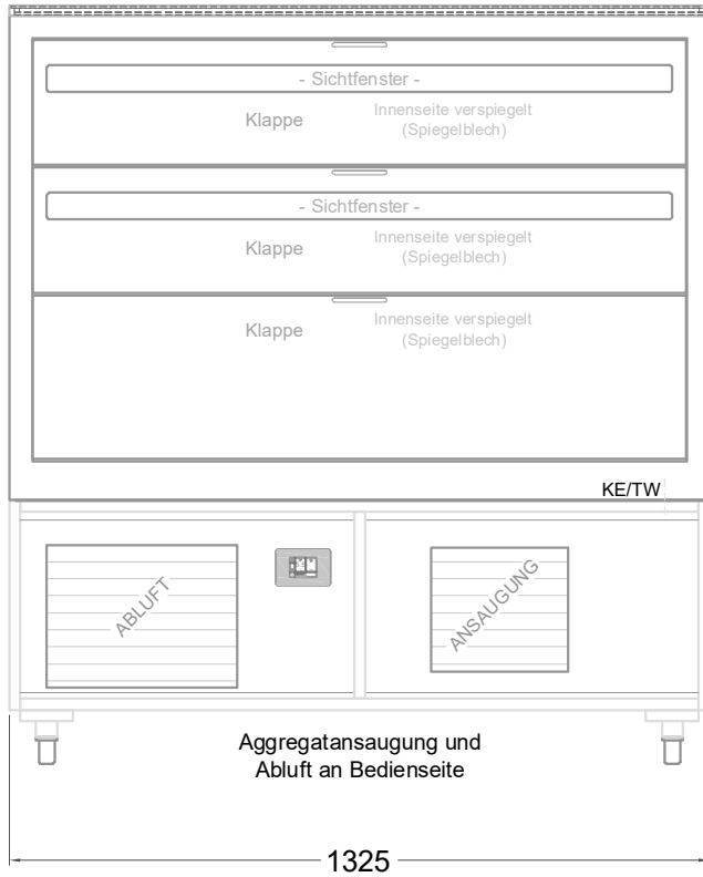
(Bedienseite)
