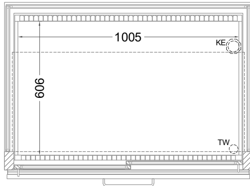
(Grundriss)
