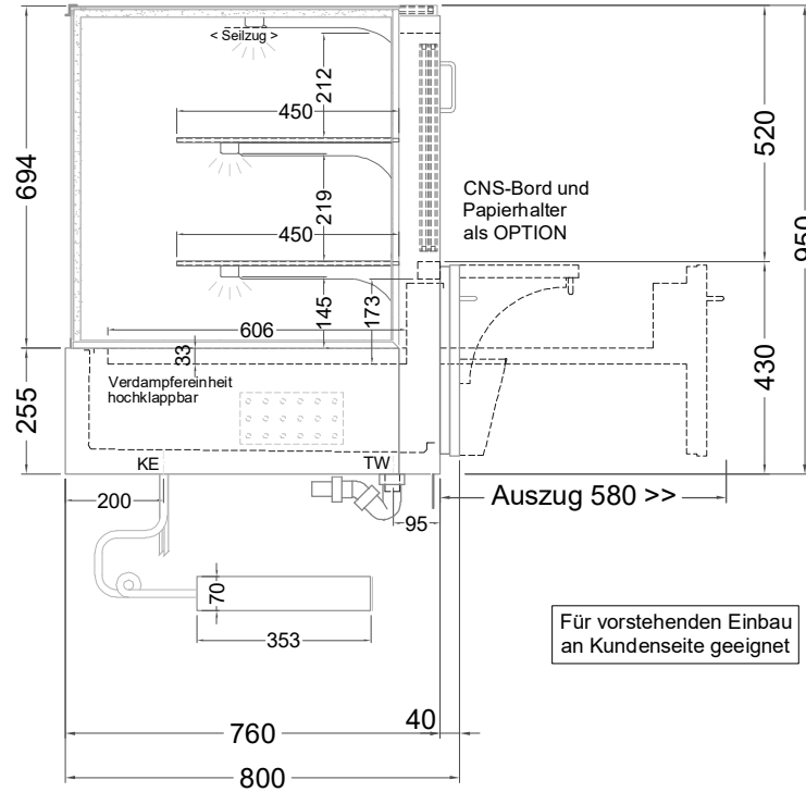
(Seitenansicht)
