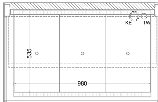
(Grundriss)
