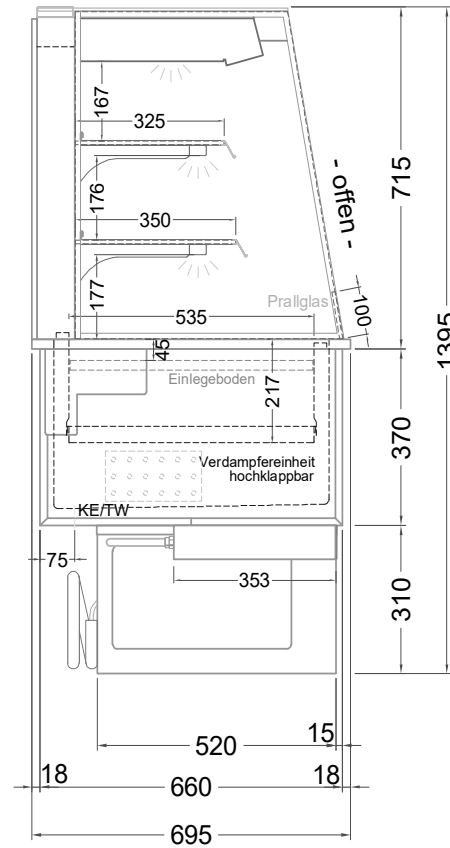
(Seitenansicht)
