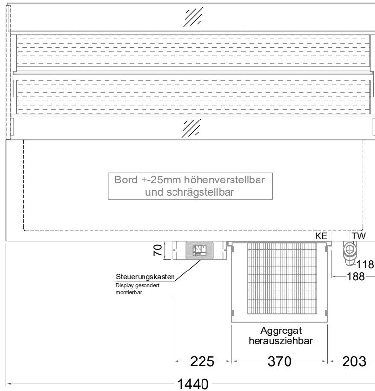
(Grundriss)
