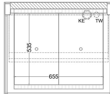
(Grundriss)
