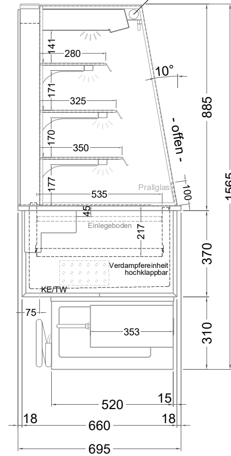
(Seitenansicht) Rollo
