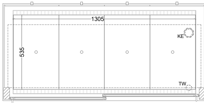
(Grundriss)
