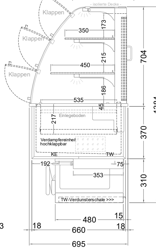
(Seitenansicht)
