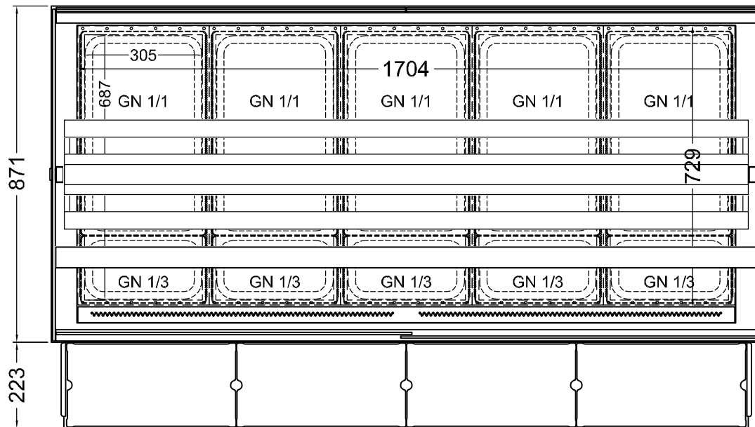
(Grundriss)
